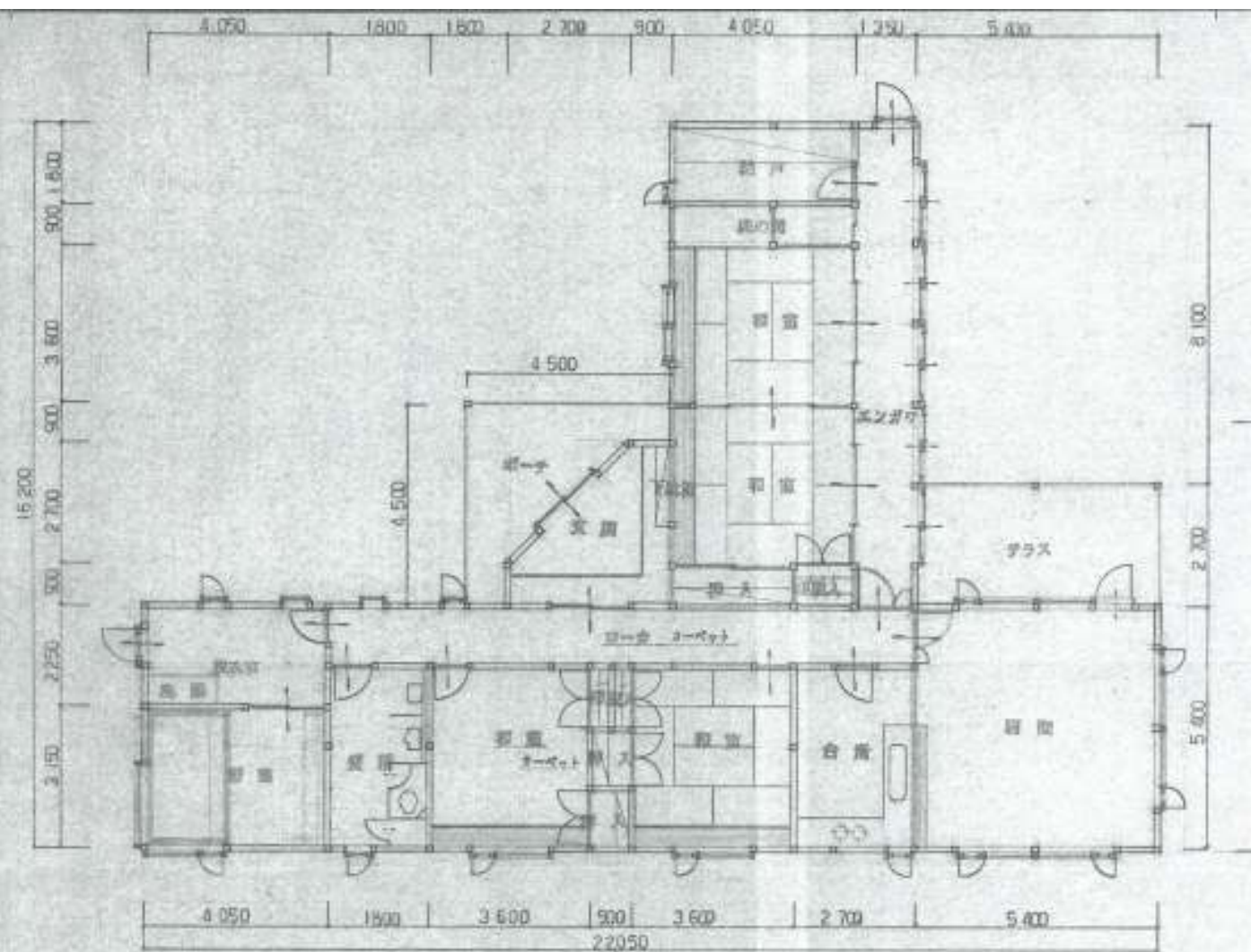
平面図 8=1/100
